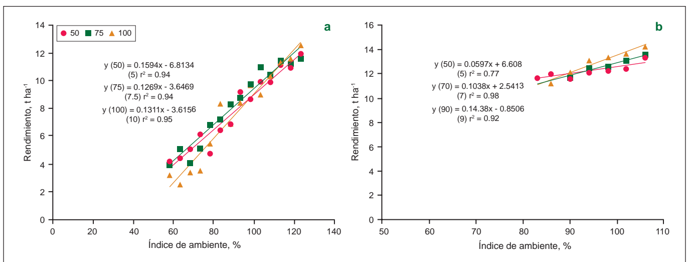
Figura 2. Rendimiento en función del índice de ambiente, para tres densidades de plantas a cosecha (miles plantas ha⁻¹) en EC, campañas 2009/10 (a; n=851), y 2010/11 (b; n=1037).
