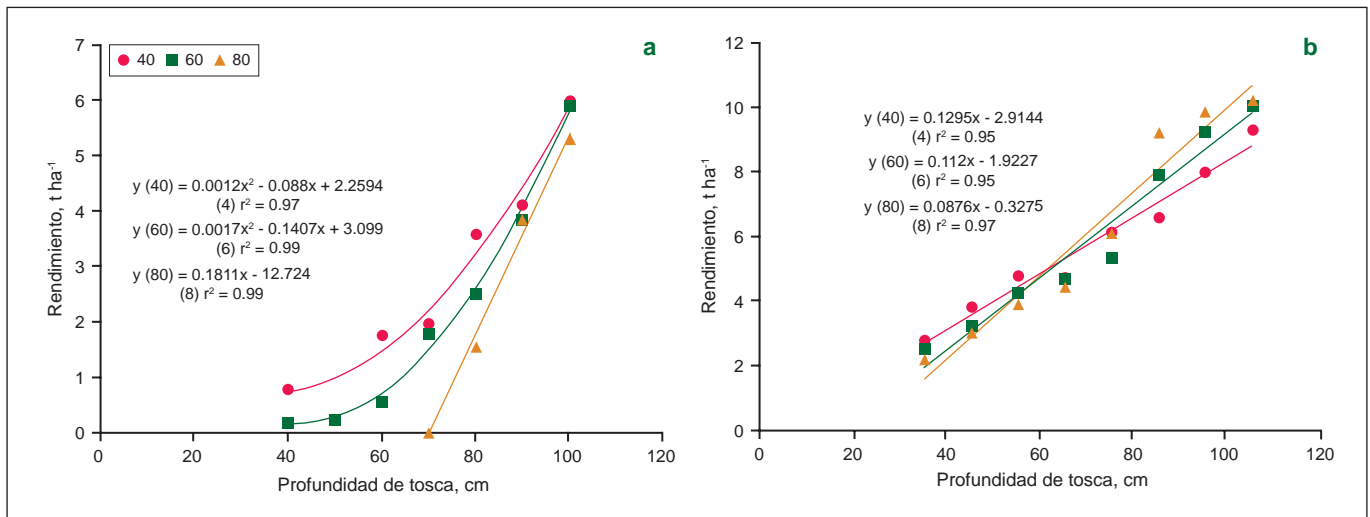
Figura 1. Rendimiento en función de la profundidad de tosca, para tres densidades de plantas a cosecha (miles plantas ha⁻¹) en TA, campañas 2009/10 (a; n=575) y 2010/11 (b; n=851).
