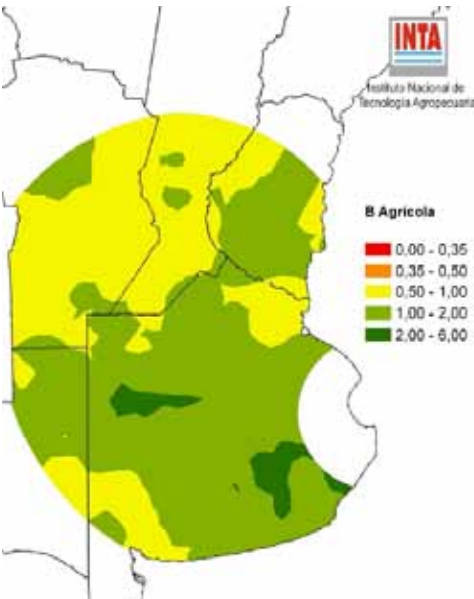
Figura 1. Mapa de valores de Boro disponible en la región pampeana (Sainz Rosas, 2013).
