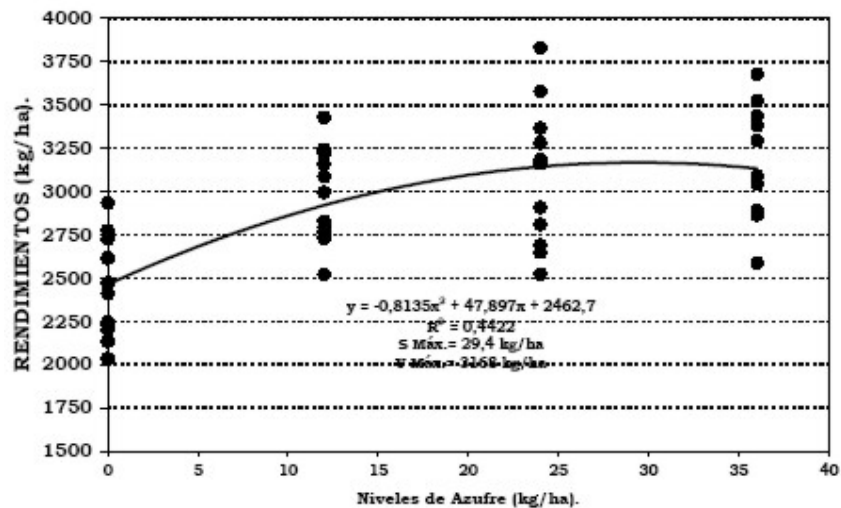
Gráfico 6. Rendimientos de soja RA 418 en función de los niveles de S residual. Bernardo de Irigoyen. 2005-06.
