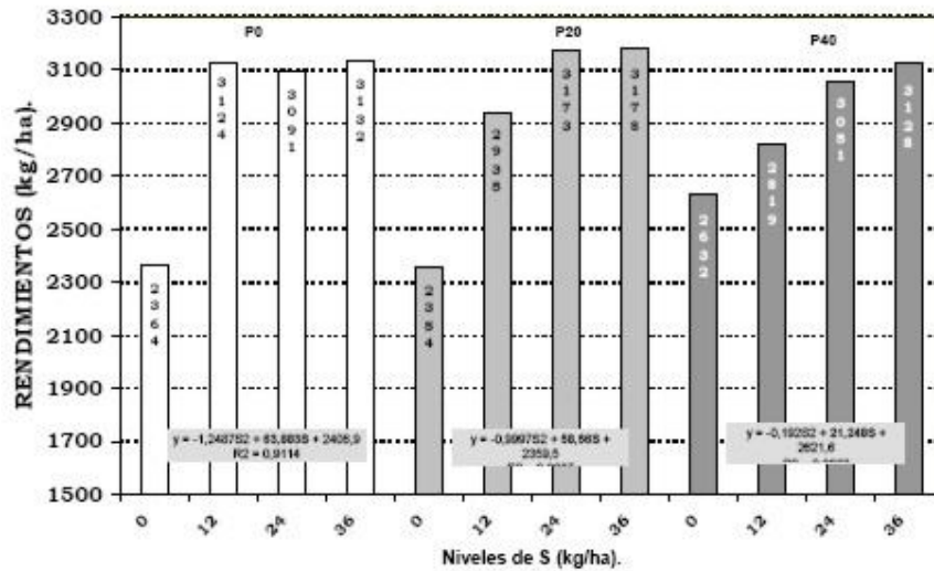
Gráfico 5. Rendimientos de soja de 1° variedad RA 418. Efectos residuales de la fertilización con P y S. Funciones de S cuadrático para cada nivel de P. Bernardo de Irigoyen, 2005-06.
